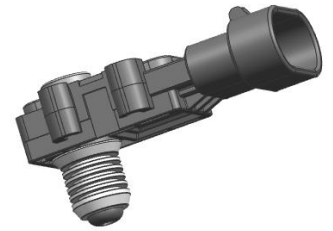
燃油蒸汽压力传感器 EVAP Pressure Sensor
